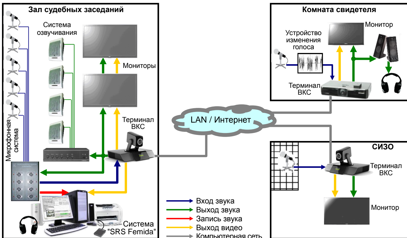
Рис.1. Компоненты системы дистанционного допроса "SRS TeleConnect"
